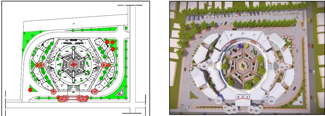
Gambar 7. Layout (Kiri) dan Siteplan (Kanan) Shopping Mall Terbuka (Sumber: penulis, 2023)
