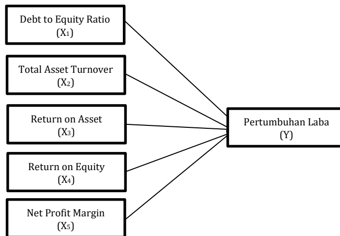
Gambar 1 Kerangka Pemikiran
