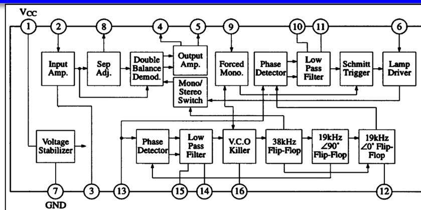
Fig. 5. AN7410N Block Diagram
