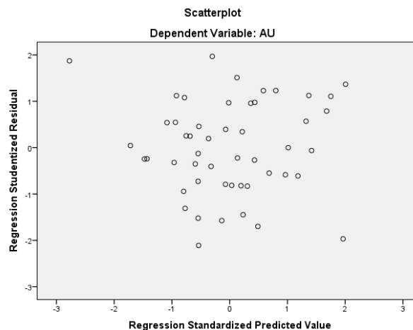
Gambar 4. Grafik scatterplot
